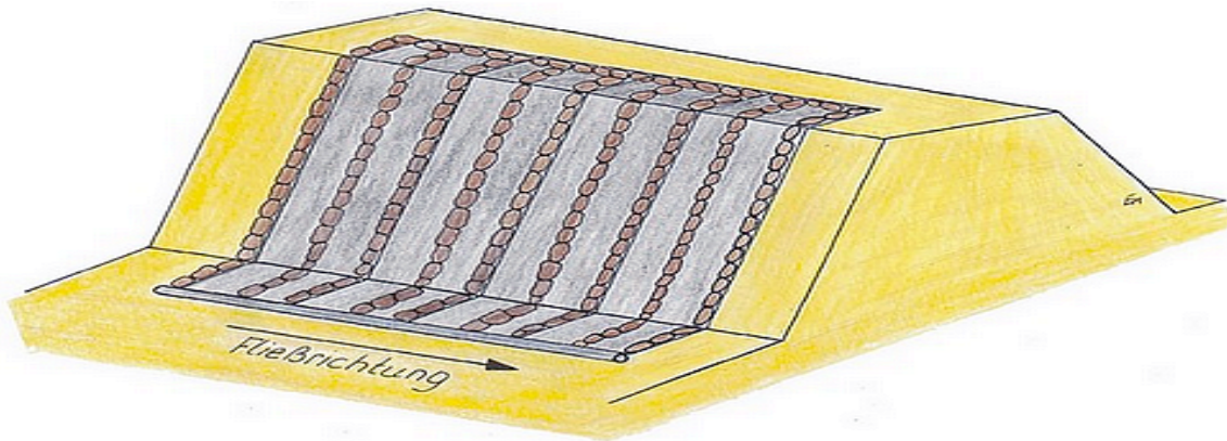
Bild 9: Skizze zur Sicherung auf der Wasserseite
