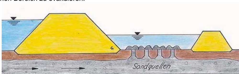
Bild 25: Funktion eines Qualmdeiches
