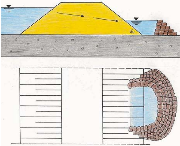
Bild 19: Prinzipskizze Quellkade
