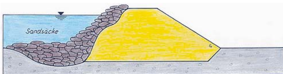
Bild 10: Sicherung der wasserseitigen Schadstelle
