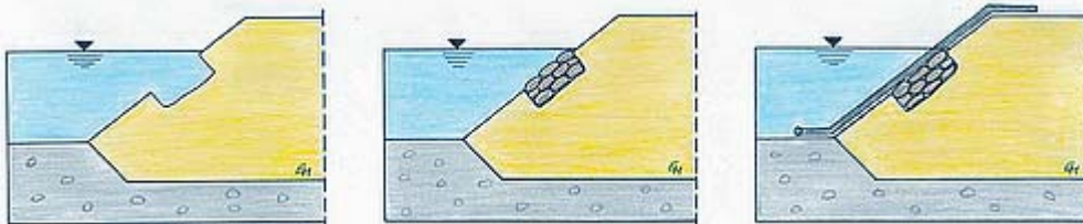
Bilder 6 bis 8: Schadensbeseitigung auf der Wasserseite
