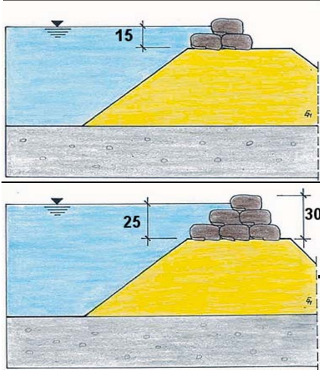
Bilder 15 u.16: Unterschiedliche Aufkadenhöhen
