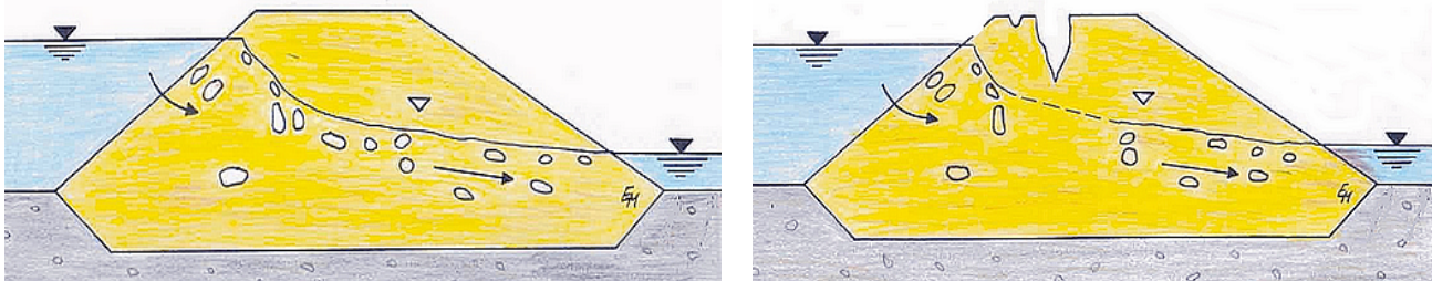
Bilder 17 und 18: Darstellung der Suffosion
