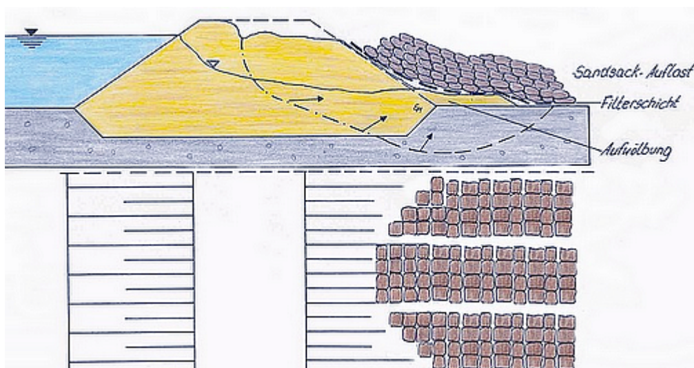
Bild 23: Prinzipskizze
