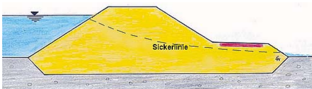
Bild 21: Herausbildung der Sickerlinie
