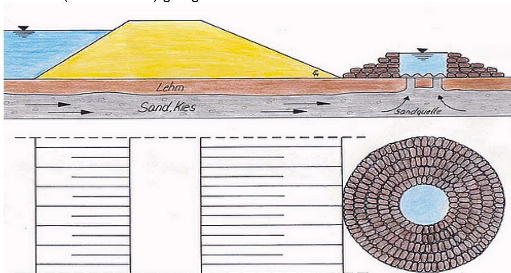
Bild 24: Prinzipskizze
