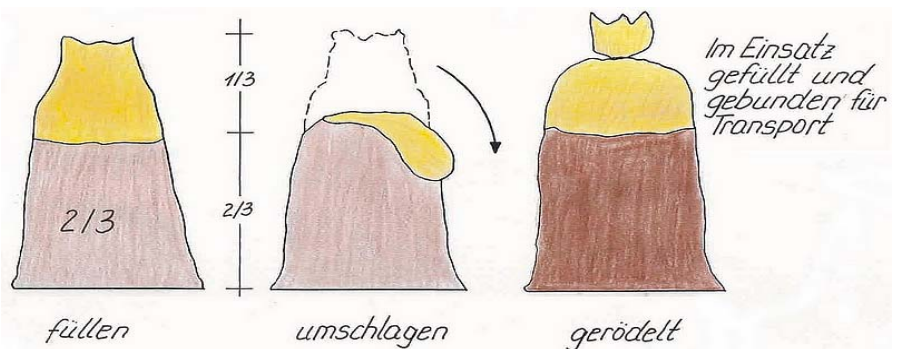
Bild 3: Füllen der Sandsäcke
