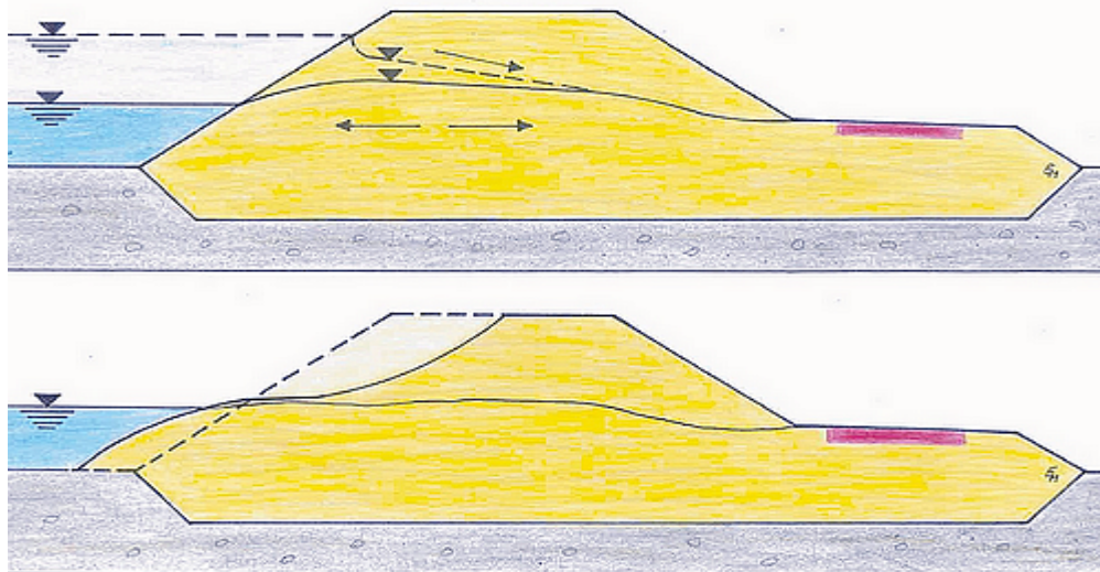
Bild 11: Umkehrung des Sickerliniengefälles
