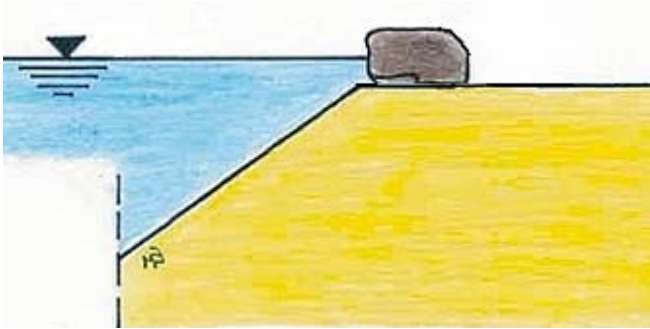
Bild 13: Verlegeart 1: Umschlagen zum Wasser
