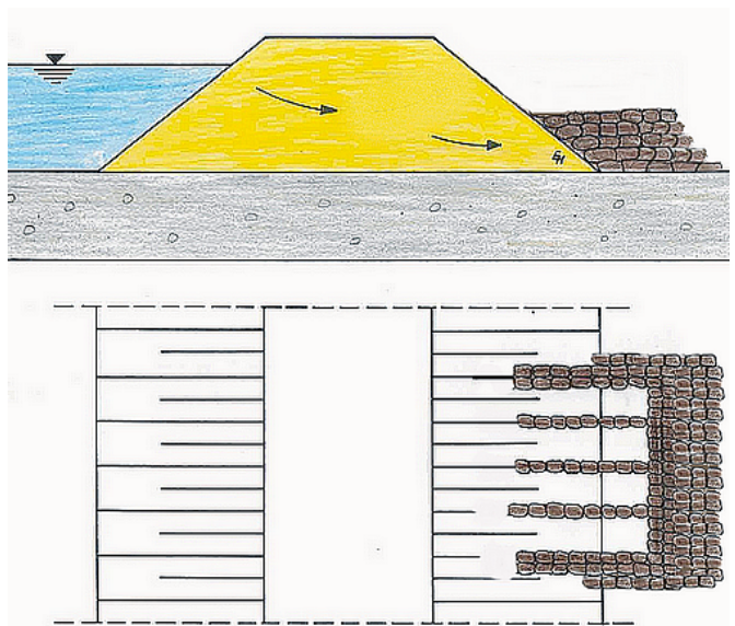
Bild 20: Prinzipskizze Kammkade
