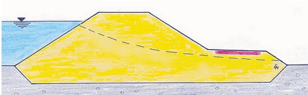
Bild 5: Ausbildung der Sickerlinie
